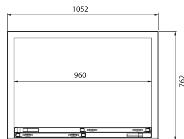
ВИД СВЕРХУ
